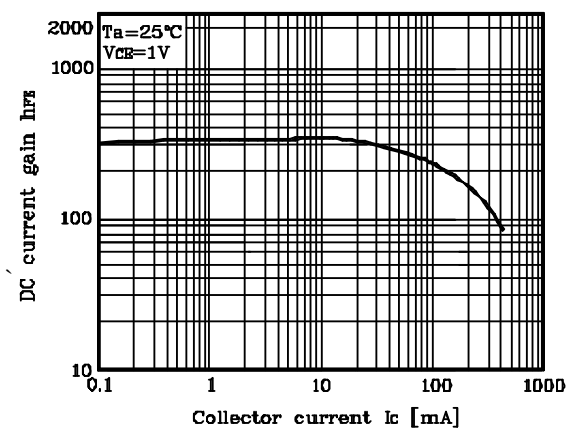
Fig. 3 h_{FE} - I_C
