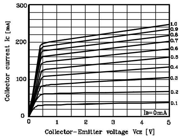
Fig. 4 I_C - V_{CE}
