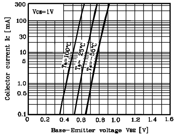
Fig. 2 I_C - V_{BE}
