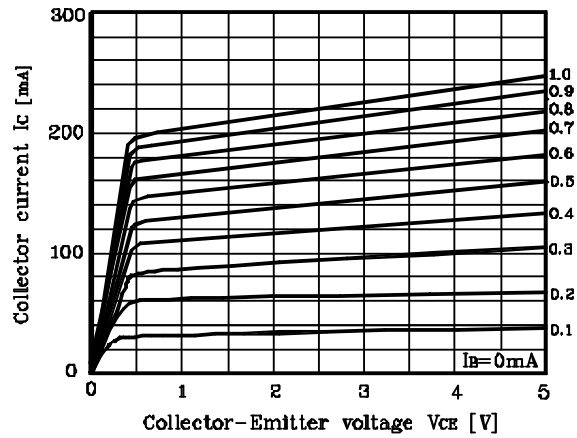
Fig. 4 I_C - V_{CE}
