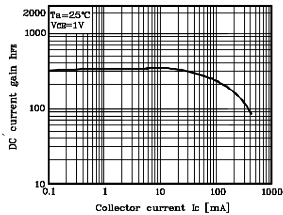
Fig. 3 h_{FE} - I_C
