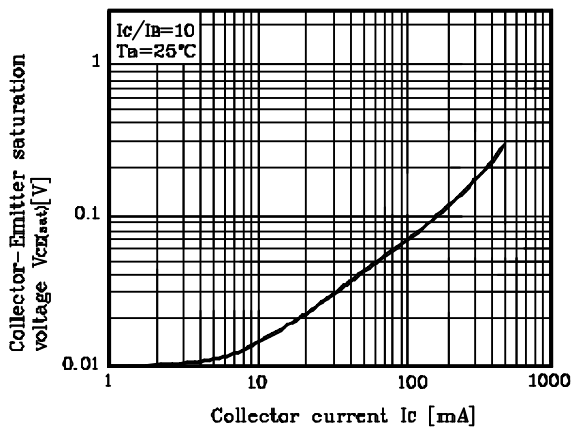
Fig. 5 V_{CE(sat)} - I_C
