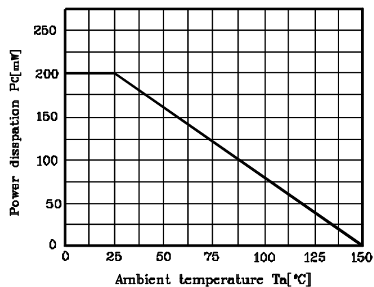
Fig. 1 P_C - T_a
