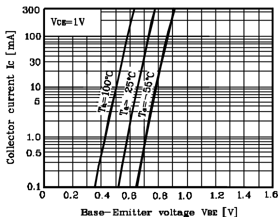
Fig. 2 I_C - V_{BE}
