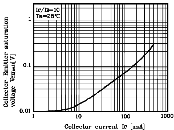
Fig. 5 V_{CE(sat)} - I_C
