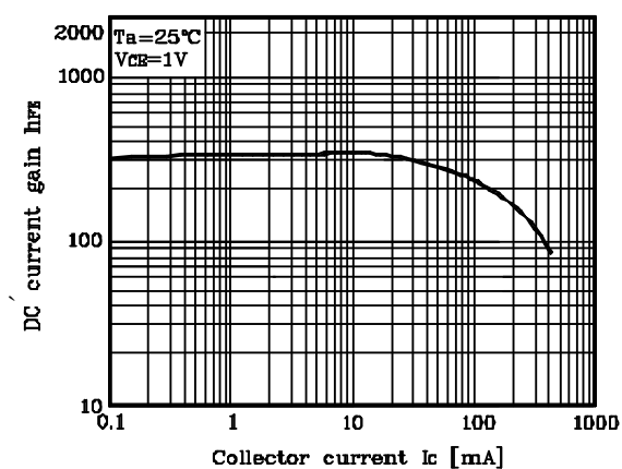
Fig. 3 h_{FE} - I_C
