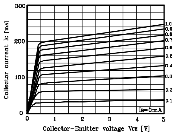
Fig. 4 I_C - V_{CE}
