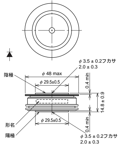
外形図
