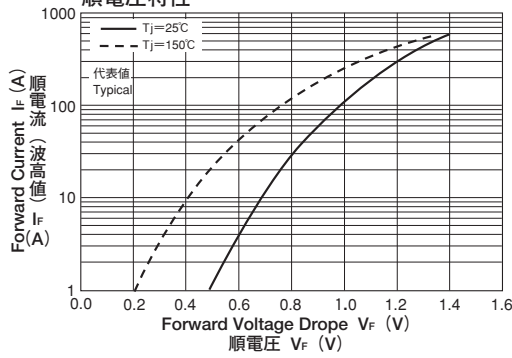
Forward Characteristics 順電圧特性
