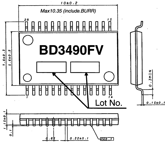
SSOP-B28 UNIT : mm (UNIT : mm)
