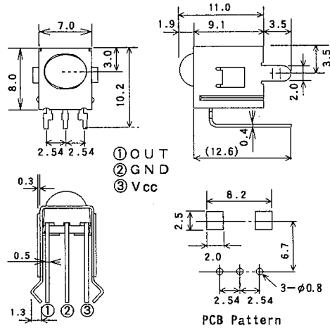
NJL63H000 UNIT : mm
