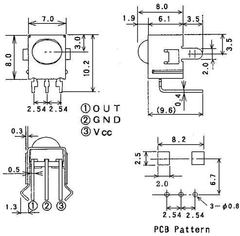
NJL62H000 UNIT : mm
