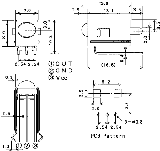
NJL64H000 UNIT : mm
