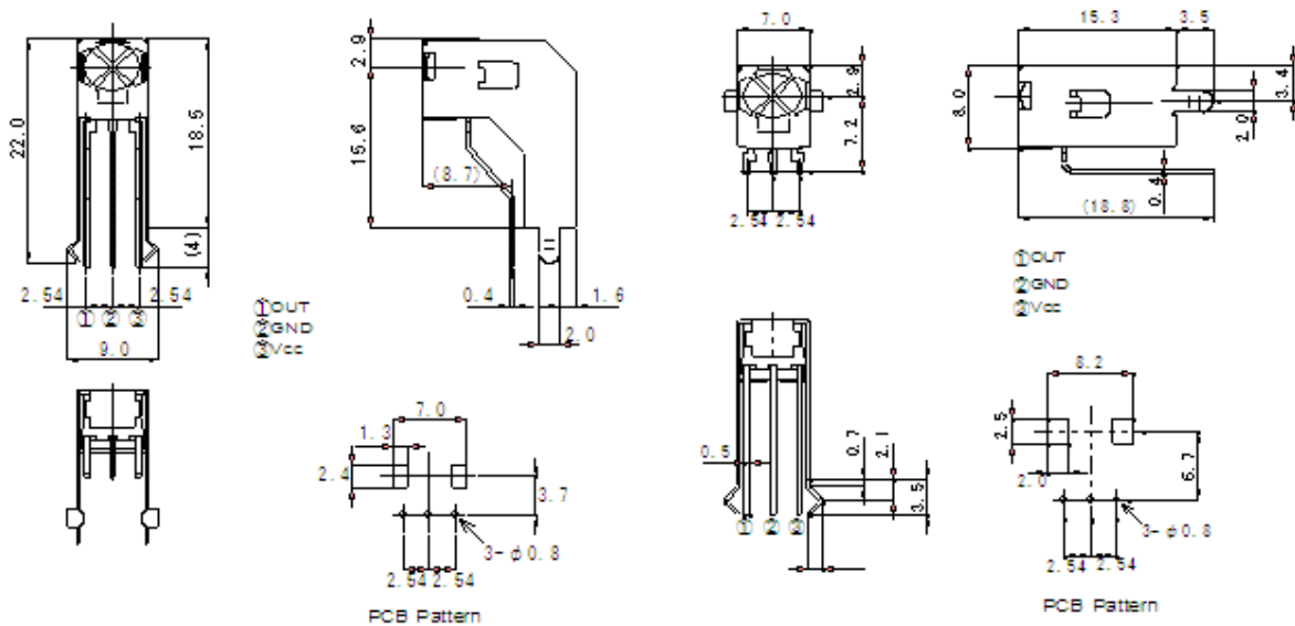
NJL35V000 UNIT:mm
