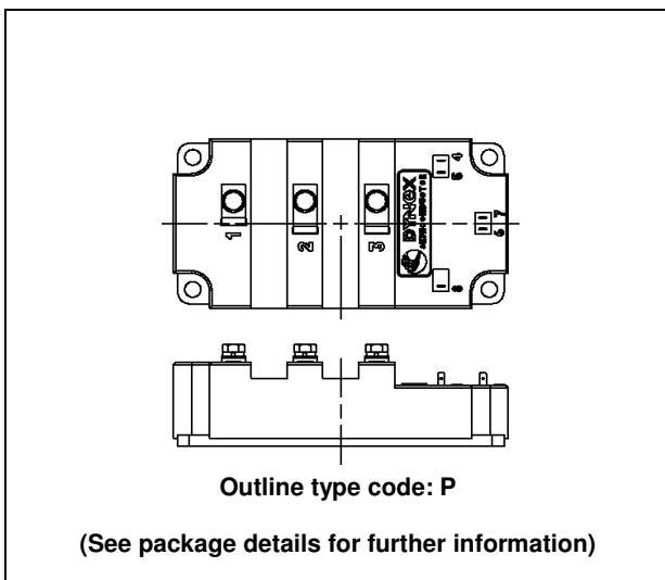
Fig. 2 Module Outline
