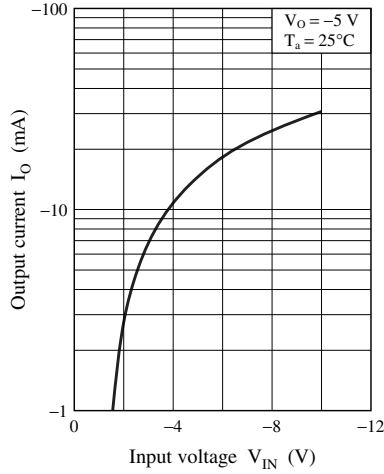
I_O - V_{IN}
