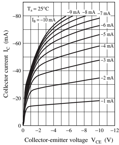
I_C - V_{CE}
