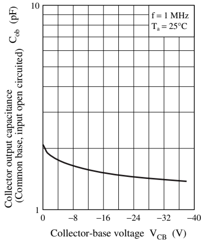
C_{ob} - V_{CB}
