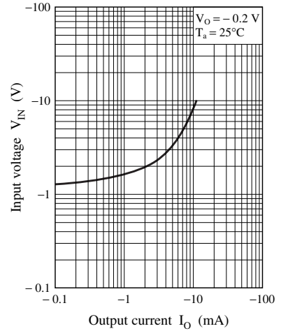
V_{IN} - I_O
