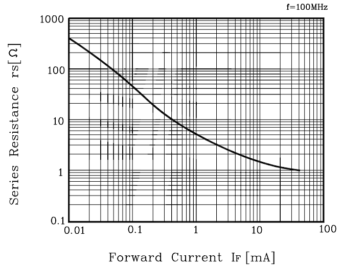
Fig. 2 r_s - I_F
