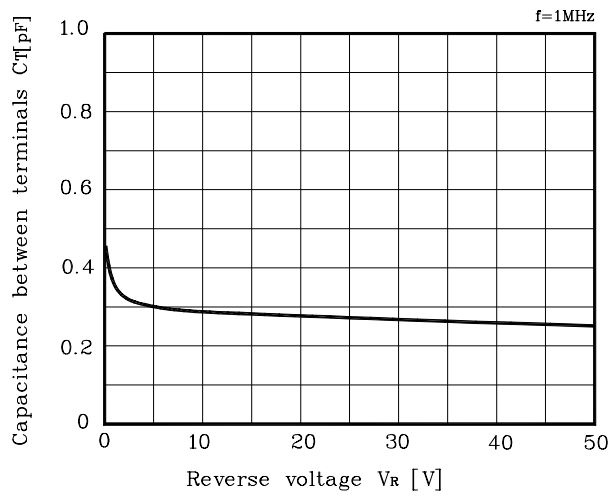
Fig. 1 C_T - V_R
