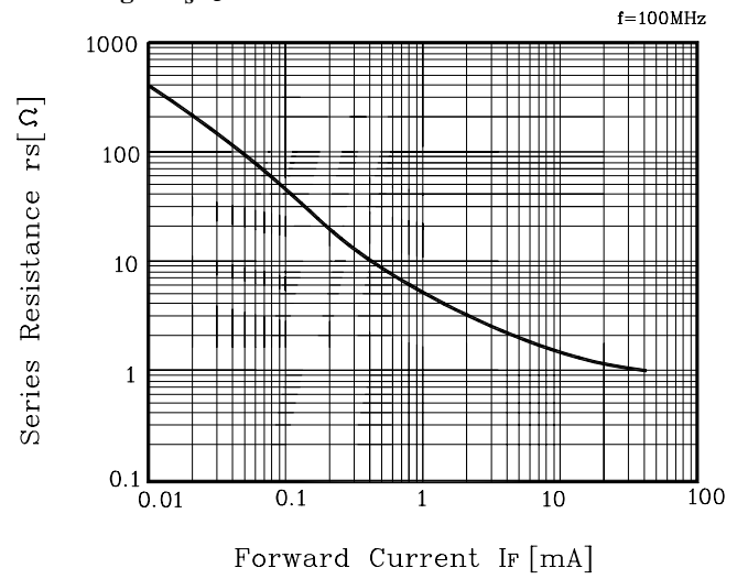
Fig. 2 r_s - I_F
