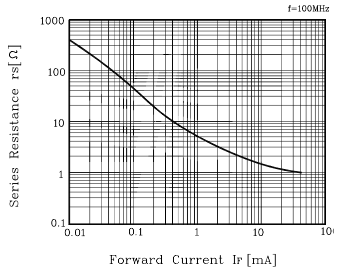
Fig. 2 r_s - I_F
