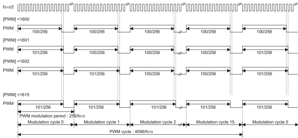
8+4 PWM Mode
