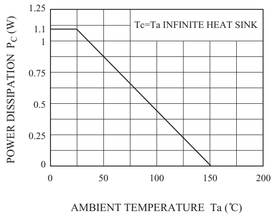
P_C - T_a
