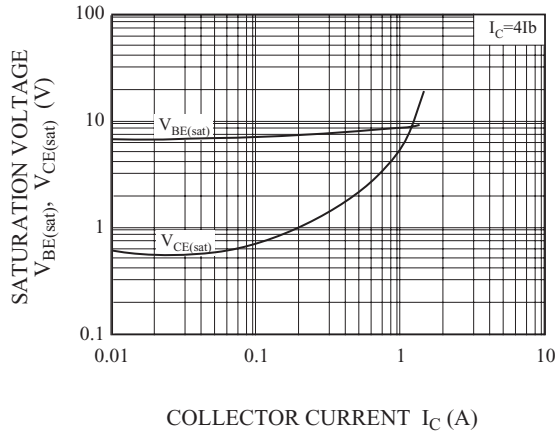
V_{CE(sat)} vs. V_{BE(sat)}
