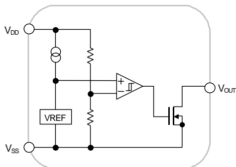
NJU7700
