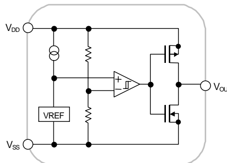
NJU7701
