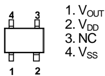
NJU7700/01F4
