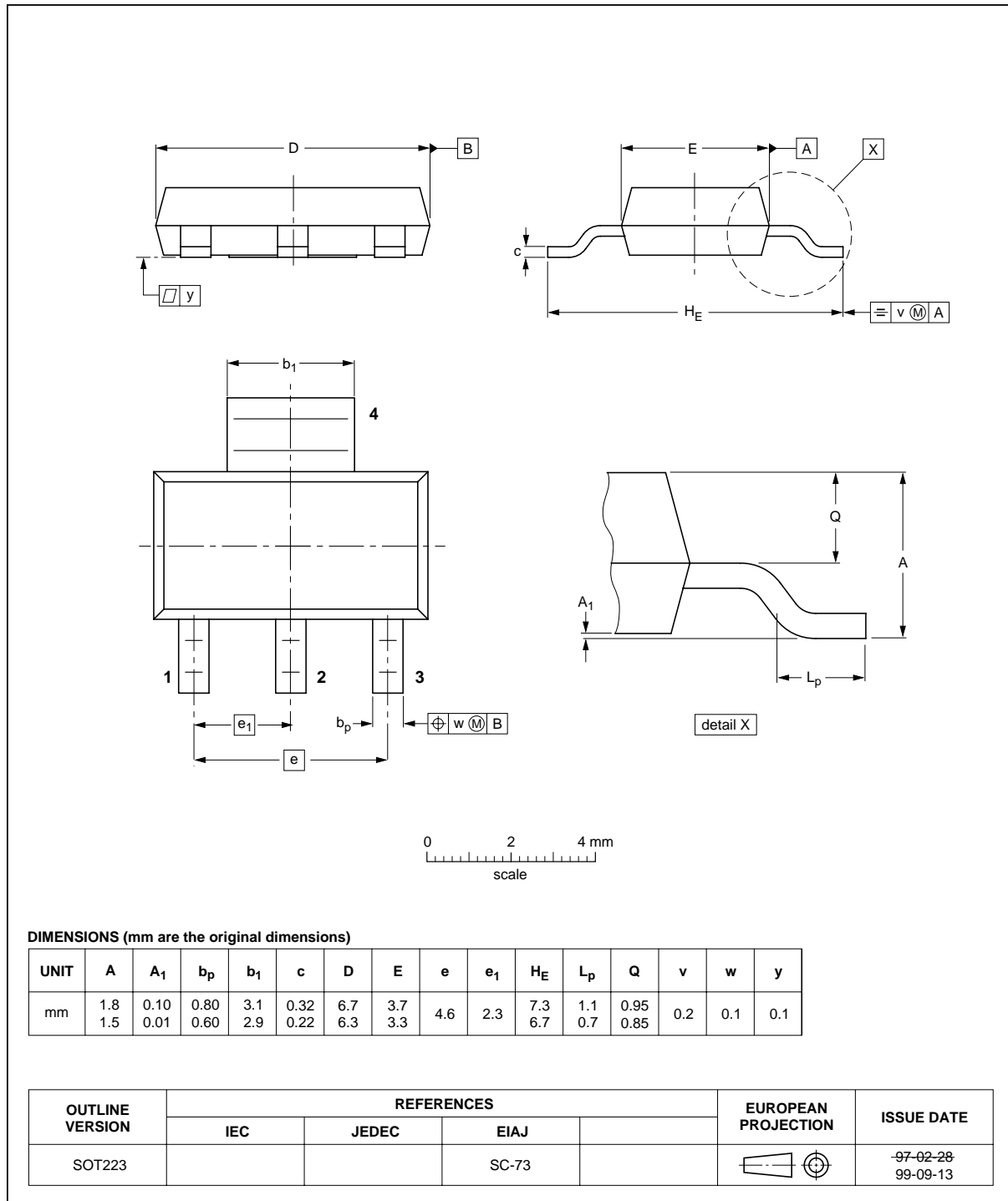
Fig 13. SOT223.
