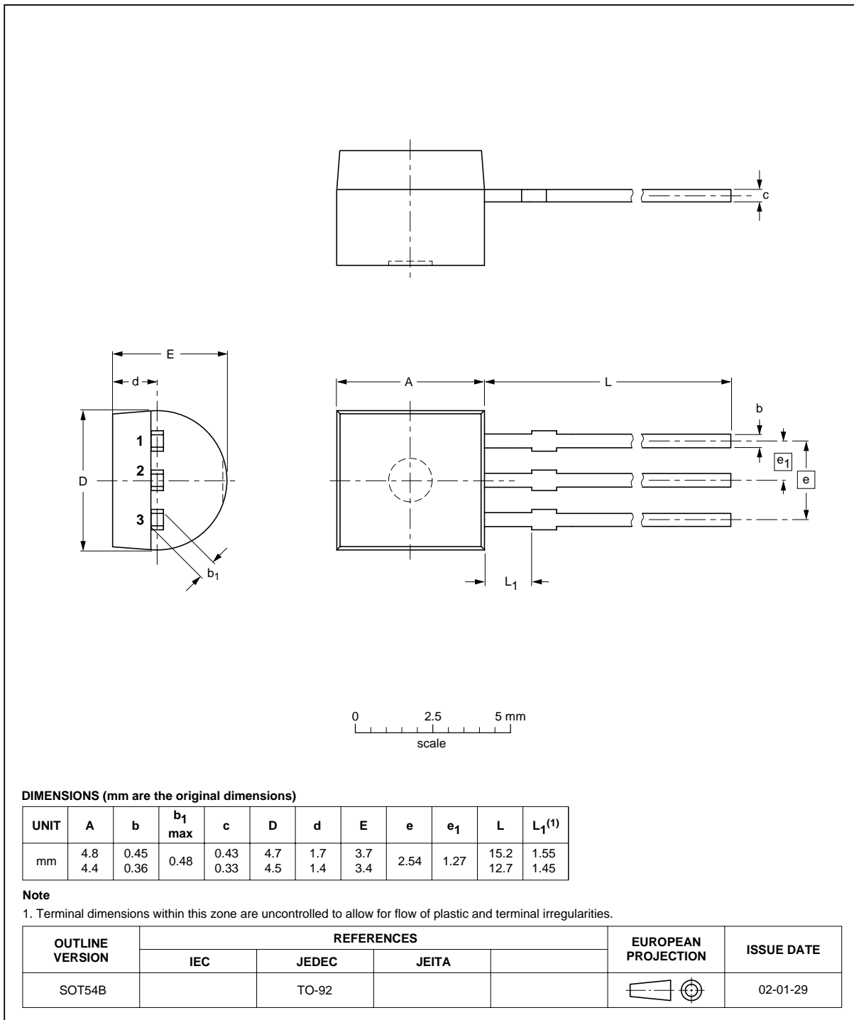
Fig 12. SOT54B (TO-92).
