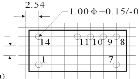
DIP 14 封装
