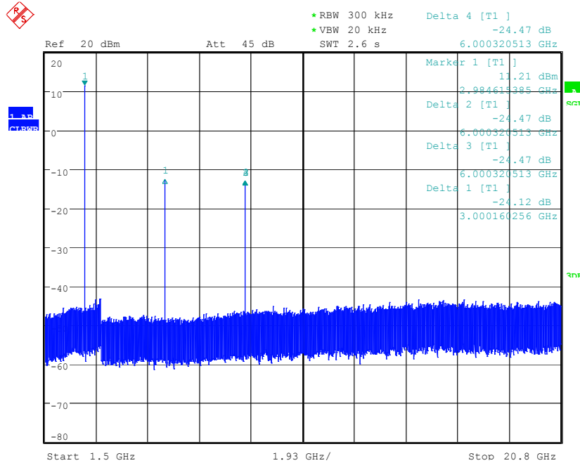
HARMONIC SUPPRESSION
