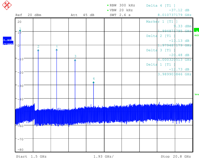
HARMONIC SUPPRESSION
