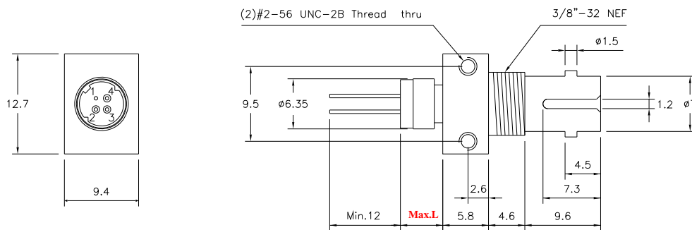
ST RECEPTACLE (DL-35XXX-TX)
