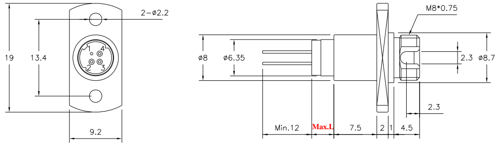
FC RECEPTACLE (DL-35XXX-FX)
