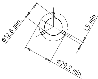
Reel hub 2:1
