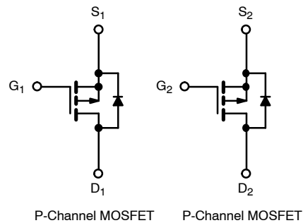
P-Channel MOSFET P-Channel MOSFET
