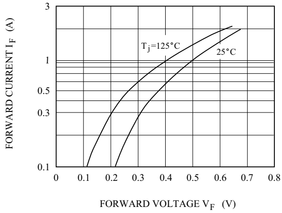
I_F - V_F
