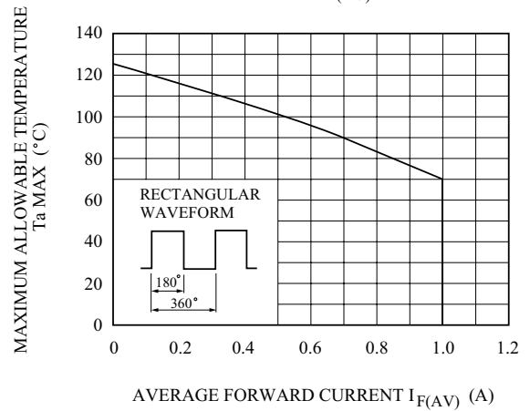
T_a - I_{F(AV)}
