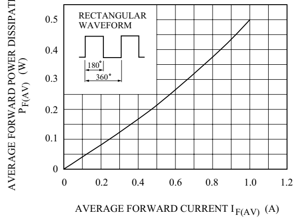
P_{F(AV)} - I_{F(AV)}
