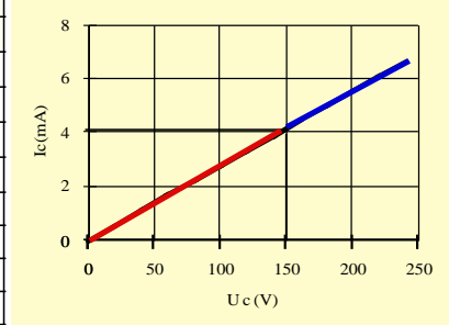
Entrée : Ic = f( Uc)
