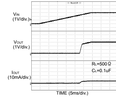
Fig.36 UVLO VIN rising
