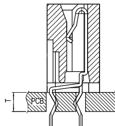
PCB ASS'Y
