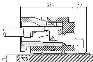
PCB ASS'Y 결함도
