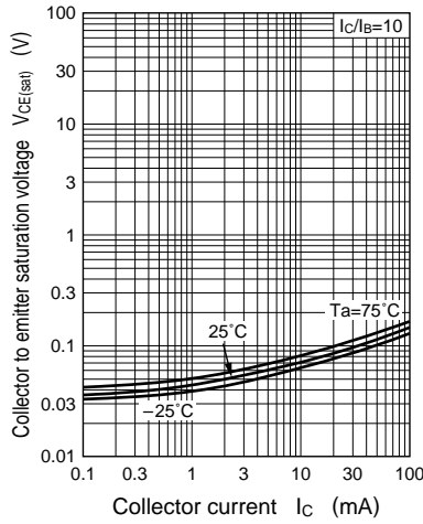
V_{CE(sat)} - I_C
