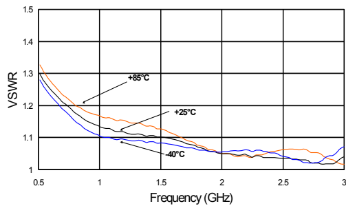
VSWR, 39 pF
