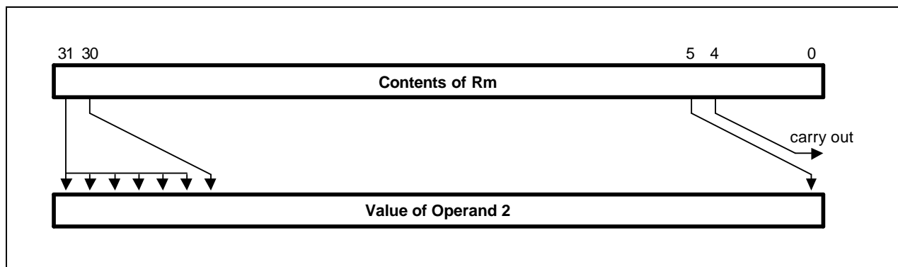
Figure 3-8. Arithmetic Shift Right
