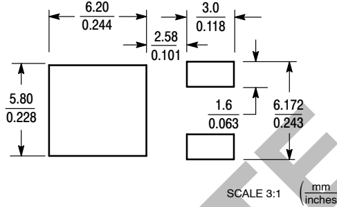
DPAK
