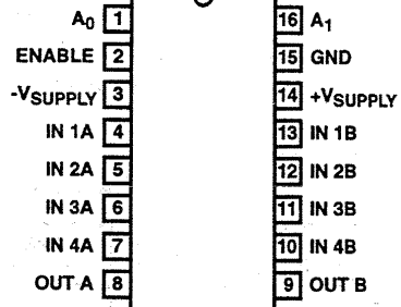
HI1-509A (CERDIP) HI3-509A (PDIP) TOP VIEW
