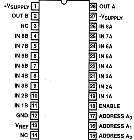
HI1-507A (CERDIP) HI3-507A (PDIP) TOP VIEW
