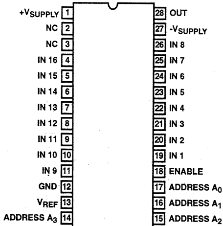
HI1-506A (CERDIP) HI3-506A (PDIP) TOP VIEW
