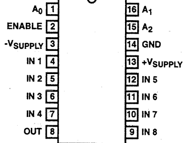
HI1-508A (CERDIP) HI3-508A (PDIP) TOP VIEW
