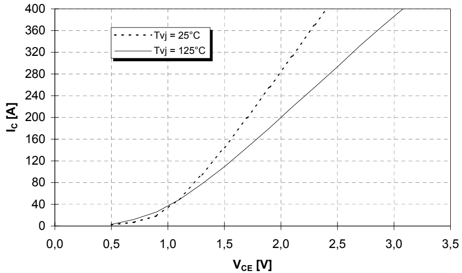
Ausgangskennlinie (typisch) output characteristic (typical)
