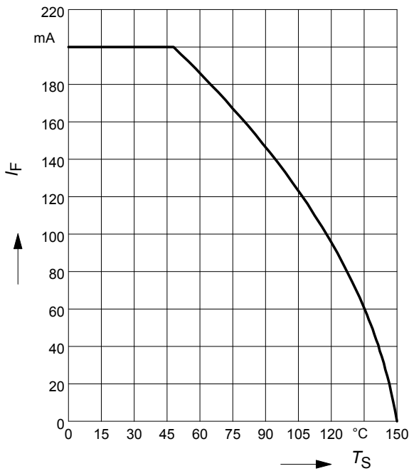
BAT54-05
