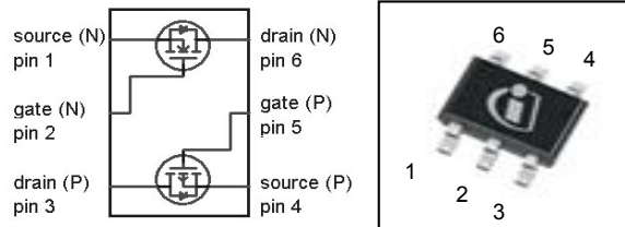
PG-SOT-363
