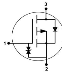
PG-SOT-23
