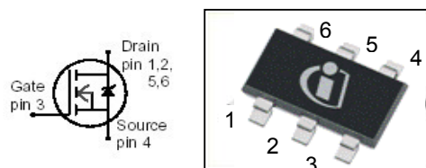
TSOP-6
