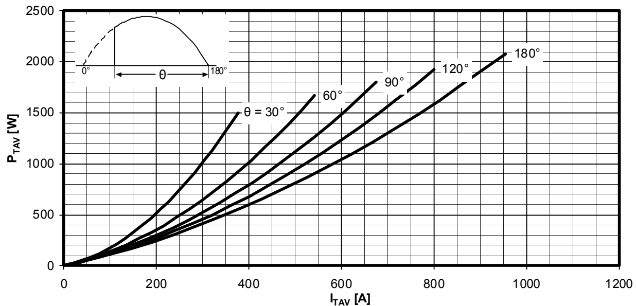
Durchlassverlustleistung / On-state power loss P_{TAV} = f(I_{TAV})
