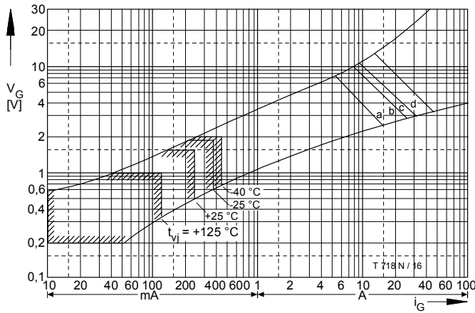
Bild / Fig. 15 Steuercharakteristik mit Zündbereichen / Gate characteristic with triggerring areas v_G = f(i_G) , V_D = 6\text{ V} Parameter: a b c d Steuerimpulsdauer / trigger puls duration t_g [ms] 10 1 0,5 0,1 Höchstzulässige Spitzensteuerverlustleistung / Max. rated peak gate power dissipation [W] 40 80 100 150
