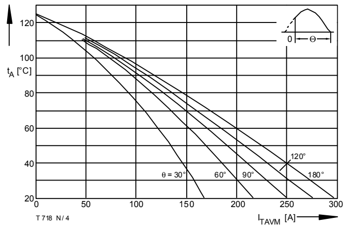
Bild / Fig. 4 Höchstzulässige Kühlmitteltemperatur / Max. allowable cooling medium temperature t_A = f(I_{TAVM}) Kühlkörper / Heatsink: K0.05F Luftseitige Kühlung / Natural air-cooling Parameter: Stromflußwinkel / Current conduction angle \theta
