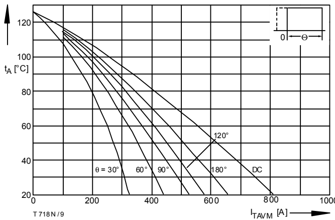
Bild / Fig. 9 Höchstzulässige Kühlmitteltemperatur / Max. allowable cooling medium temperature t_A = f(I_{TAVM}) Verstärkte Luftkühlung / forced air cooling Kühlkörper / Heatsink: K0.55F, V_L = 120 l/s Parameter: Stromflußwinkel / Current conduction angle \theta
