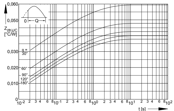
Bild / Fig. 18 Transienter innerer Wärmewiderstand / Transient thermal impedance Z_{thJC} = f(t) Beidseitige Kühlung / Two-sided cooling Parameter: Stromflußwinkel / current conduction angle q
