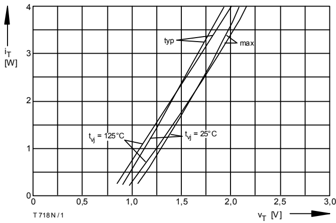
Bild / Fig. 1 Durchlaßkennlinien / On-state characteristics i_T = f(v_T)
