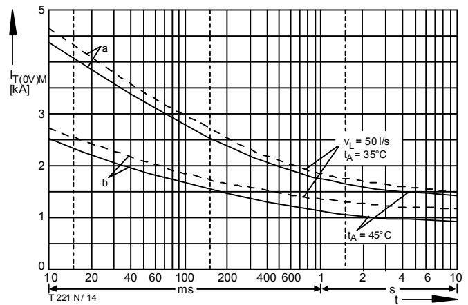
Bild / Fig. 14 Grenzstrom / Max. overload on-state current I_{T(OV)M} = f(t) , v_{RM} = 0,8 V_{RRM} ----- Luftselbstkühlung / Natural air-cooling, t_A = 45^\circ C ----- Verstärkte Luftkühlung / Forced air-cooling, t_A = 35^\circ C Kühlkörper / Heatsink: K0.55-FB54-A, V_L = 50 l/s Belastung aus / Surge current occurs: a - Leerlauf / No-load conditions b - Betrieb mit Dauergrenzstrom / During operation at max. average on-state current I_{TAVM}
