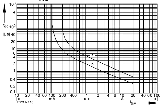
Bild / Fig. 16 Zündverzögerung / Gate controlled delay time t_{gd} = f(i_{GM}) t_{vj} = 25^\circ C , di_G/dt = i_{GM}/1\mu s a - Maximaler Verlauf / Limiting characteristic b - Typischer Verlauf / Typical characteristic
