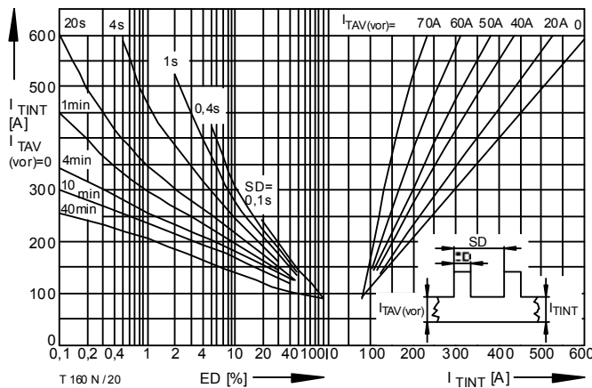
Bild / Fig. 20 Höchstzulässiger Durchlaßstrom bei Aussetzbetrieb / Max. allowable on-state current at intermittent operation I_{TINT} = f(ED) Luftselbstkühlung / Natural air-cooling, t_A = 45^\circ\text{C} Kühlkörper / Heatsink: K0.55-FB54-A Parameter: Spieldauer / Cycle duration SD Vorlaststrom / Pre-load current I_{TAV(vor)}
