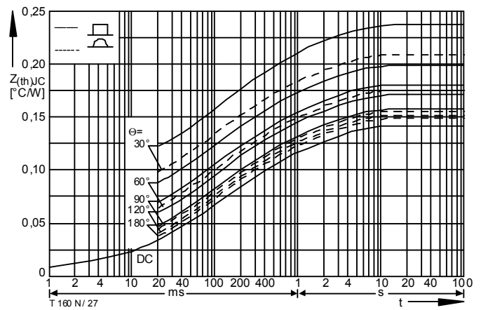
Bild / Fig. 27 Transienter inerer Wärmewiderstand / Transient thermal impedance Z_{thJC} = f(t) Parameter: Stromfußwinkel / current conduction angle \theta
