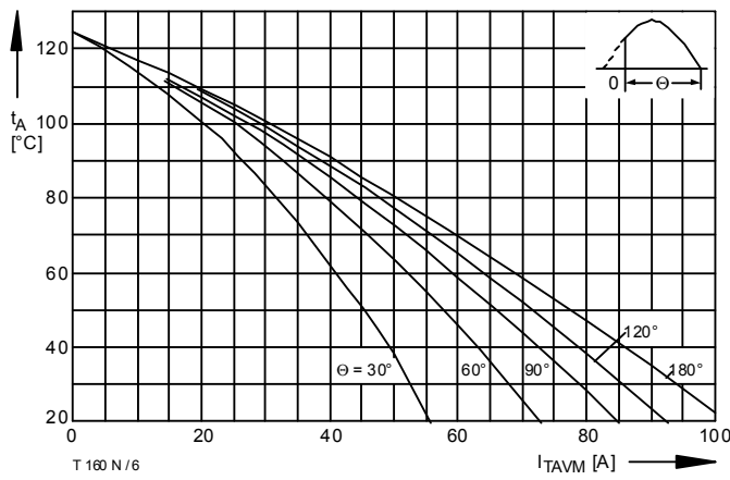
Bild / Fig. 6 Höchstzulässige Kühlmitteltemperatur / Max. allowable cooling medium temperature t_A = f(I_{TAVM}) Luftselbstkühlung / Natural air-cooling Kühlkörper / Heatsink: K0.55-M12-A Parameter: Stromflußwinkel / Current conduction angle \theta
