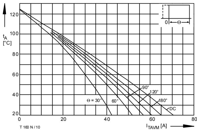
Bild / Fig. 10 Höchstzulässige Kühlmitteltemperatur / Max. allowable cooling medium temperature t_A = f(I_{TAVM}) Luftselbstkühlung / Natural air-cooling Kühlkörper / Heatsink: K1.1-M12-A Parameter: Stromflußwinkel / Current conduction angle \theta
