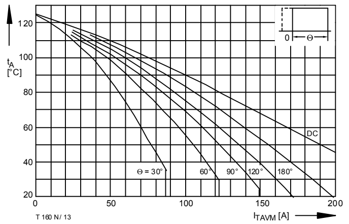
Bild / Fig. 13 Höchstzulässige Kühlmitteltemperatur / Max. allowable cooling medium temperatur t_A = f(I_{TAVM}) Verstärkte Luftkühlung / Forced air-cooling, Kühlkörper / Heatsink: K0.55-M12-A, V_L = 50 l/s Parameter: Stromflußwinkel / Current conduction angle \theta
