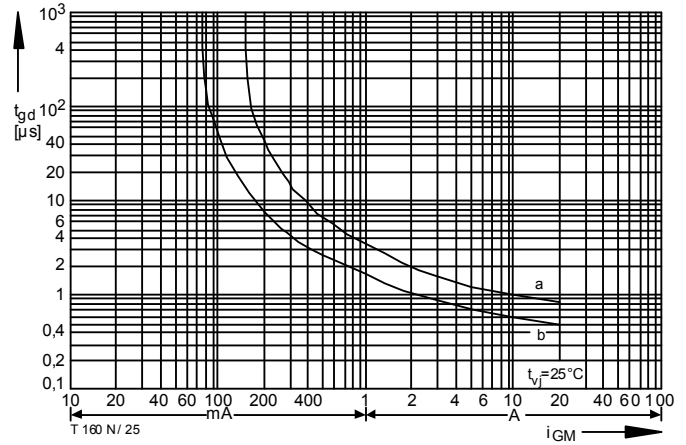
Bild / Fig. 25 Zündverzögerung / Gate controlled delay time t_{gd} = f(i_{GM}) t_{vj} = 25\text{ °C} , di_G/dt = i_{GM}/1\mu\text{s} a - Maximaler Verlauf / Limiting characteristic b - Typischer Verlauf / Typical characteristic
