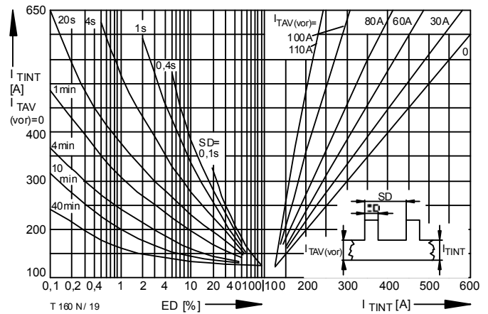
Bild / Fig. 19 Höchstzulässiger Durchlaßstrom bei Aussetzbetrieb / Max. allowable on-state current at intermittent operation I_{TINT} = f(ED) Verstärkte Luftkühlung / Forced air-cooling, t_A = 35^\circ\text{C} , V_L = 30 \text{ l/s} Kühlkörper / Heatsink: K1.1-M12-A Parameter: Spieldauer / Cycle duration SD Vorlaststrom / Pre-load current I_{TAV(vor)}
