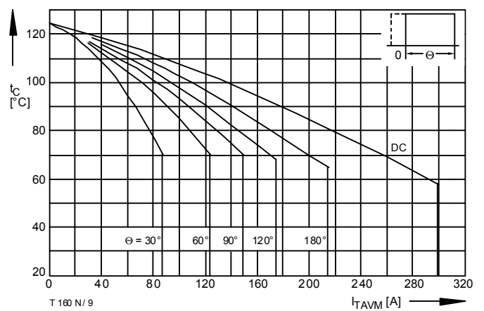
Bild / Fig. 9 Höchstzulässige Gehäusetemperatur / Max. allowable case temperature t_C = f(I_{TAVM}) Parameter: Stromflußwinkel / Current conduction angle \theta
