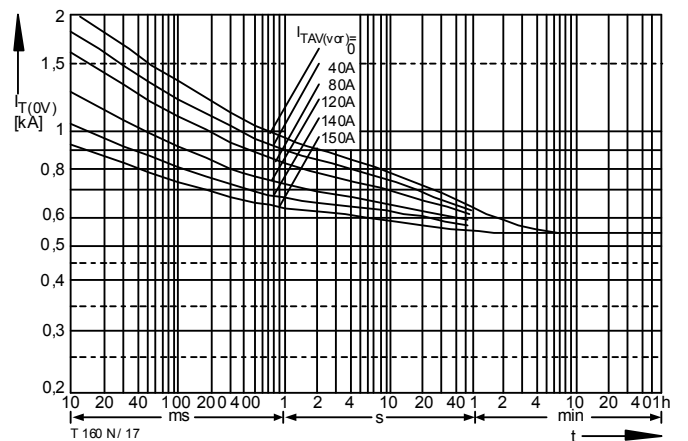
Bild / Fig. 15 Überstrom / Overload on-state current I_{T(OV)} = f(t) Verstärkte Luftkühlung / Forced air-cooling, t_A = 35^\circ\text{C} Kühlkörper / Heatsink: K0.55-M12-A, V_L = 50 l/s Parameter: Vorlaststrom / Pre-load current I_{TAV(vor)}
