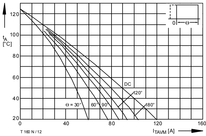
Bild / Fig. 12 Höchstzulässige Kühlmitteltemperatur / Max. allowable cooling medium temperatur t_A = f(I_{TAVM}) Luftselbstkühlung / Natural air-cooling Kühlkörper / Heatsink: K0.55-M12-A Parameter: Stromflußwinkel / Current conduction angle \theta
