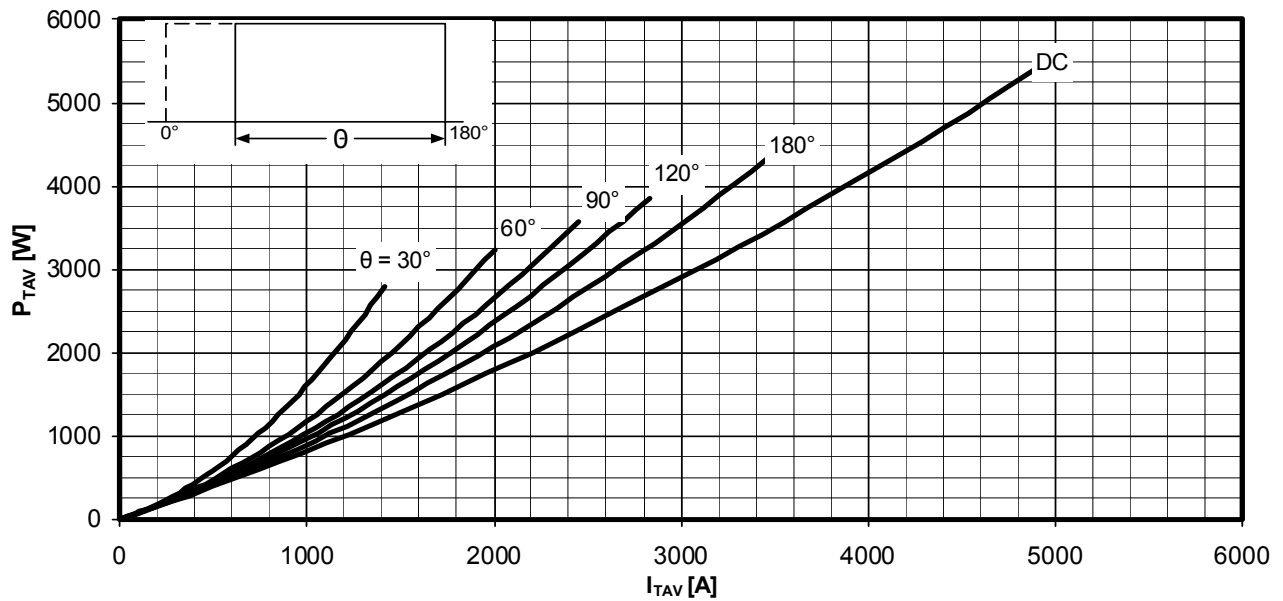
Durchlassverlustleistung / On-state power loss P_{TAV} = f(I_{TAV})
