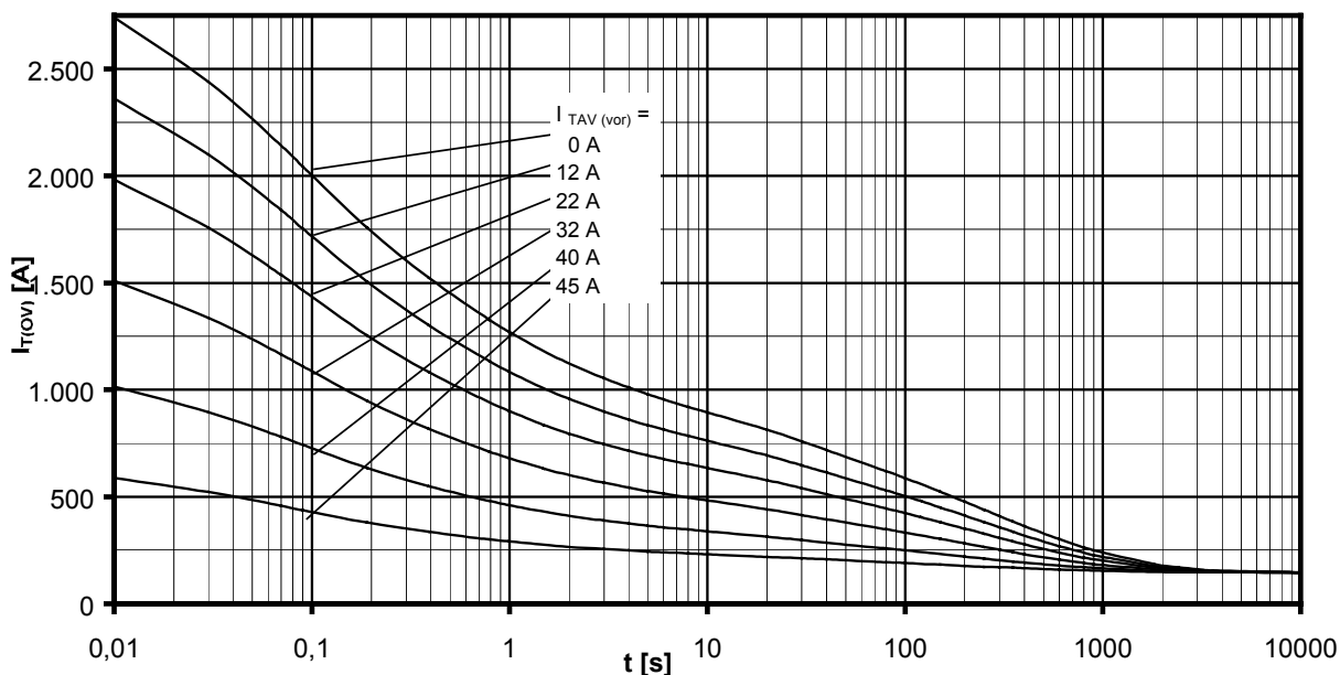
Überstrom je Zweig / Overload on-state current I_{T(OV)}
