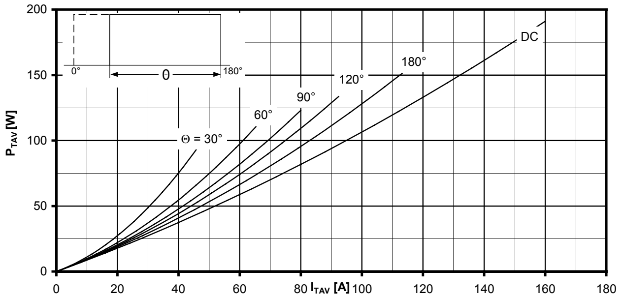
Durchlassverlustleistung je Zweig / On-state power loss per arm P_{TAV} = f(I_{TAV}) Rechteckförmiger Strom / Rectangular current Strombelastung je Zweig / Current load per arm Parameter: Stromflußwinkel / Current conduction angle \Theta
