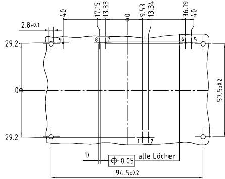
Leiterplatten-Lochbild / PCB drillhole pattern
