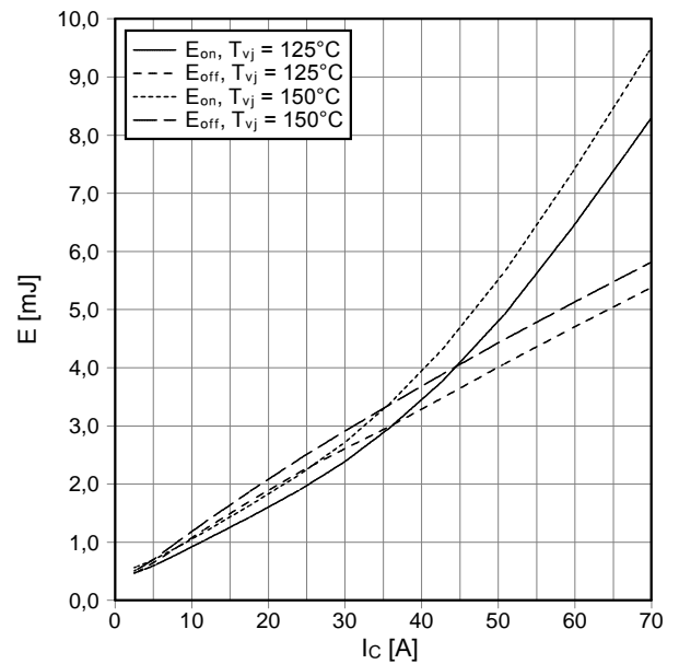
Schaltverluste IGBT-Wechselr. (typisch) switching losses IGBT-inverter (typical) E_{on} = f(I_c) , E_{off} = f(I_c) V_{GE} = \pm 15\text{ V} , R_{Gon} = 12\ \Omega , R_{Goff} = 12\ \Omega , V_{CE} = 600\text{ V}
