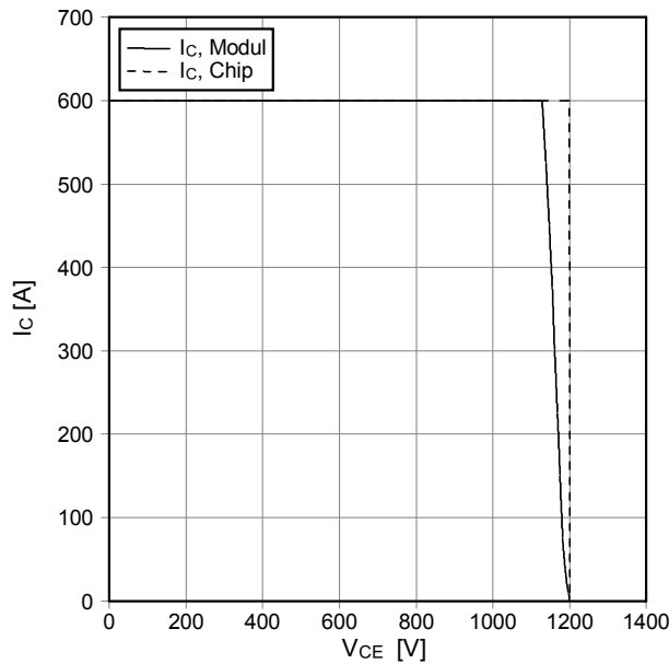
Sicherer Rückwärts-Arbeitsbereich IGBT-Wr. (RBSOA) reverse bias safe operating area IGBT-inv. (RBSOA) I_c = f(V_{CE}) V_{GE} = \pm 15\text{ V}, R_{Goff} = 0.75\ \Omega, T_{vj} = 150^\circ\text{C}
