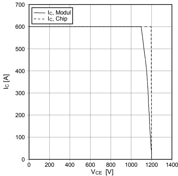
Sicherer Rückwärts-Arbeitsbereich IGBT-Wr. (RBSOA) reverse bias safe operating area IGBT-inv. (RBSOA) I_c = f(V_{CE}) V_{GE} = \pm 15\text{ V} , R_{Goff} = 0.82\ \Omega , T_{vj} = 150^\circ\text{C}
