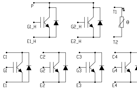
Schaltbild
