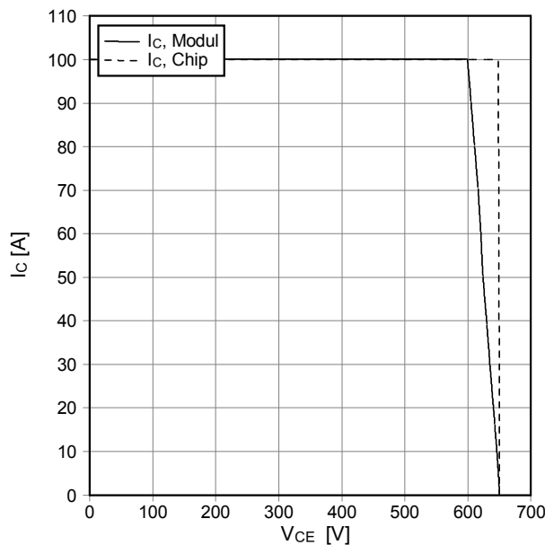
Sicherer Rückwärts-Arbeitsbereich IGBT-Wr. (RBSOA) reverse bias safe operating area IGBT-inv. (RBSOA) I_c = f(V_{CE}) V_{GE} = \pm 15\text{ V}, R_{Goff} = 6.8\ \Omega, T_{vj} = 150^\circ\text{C}
